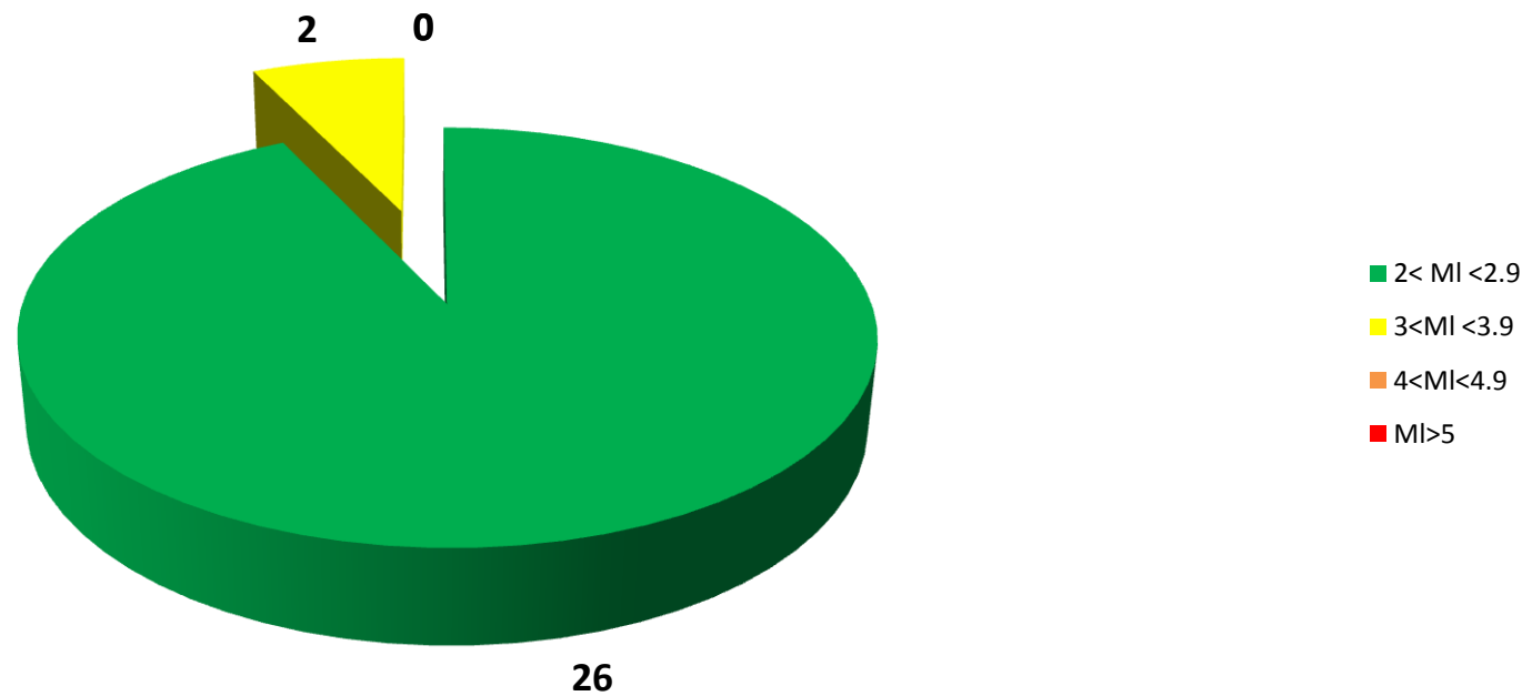
Numero sismi con Magnitudo > 2 in areale Sicilia - 1 Maggio - 31 Maggio 2014 totale di eventi 28
