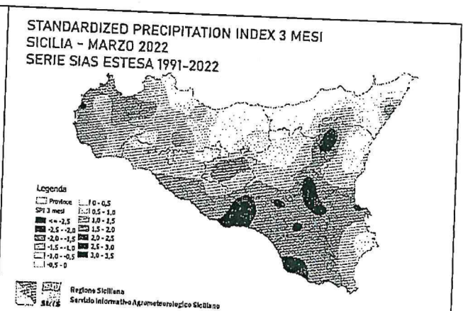
Mappa SPI 3 mesi - Marzo 2022
