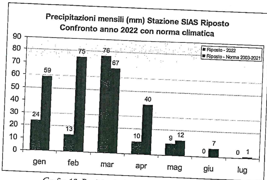
Grafico 12: Precipitazioni mensili stazione SIAS Riposto
