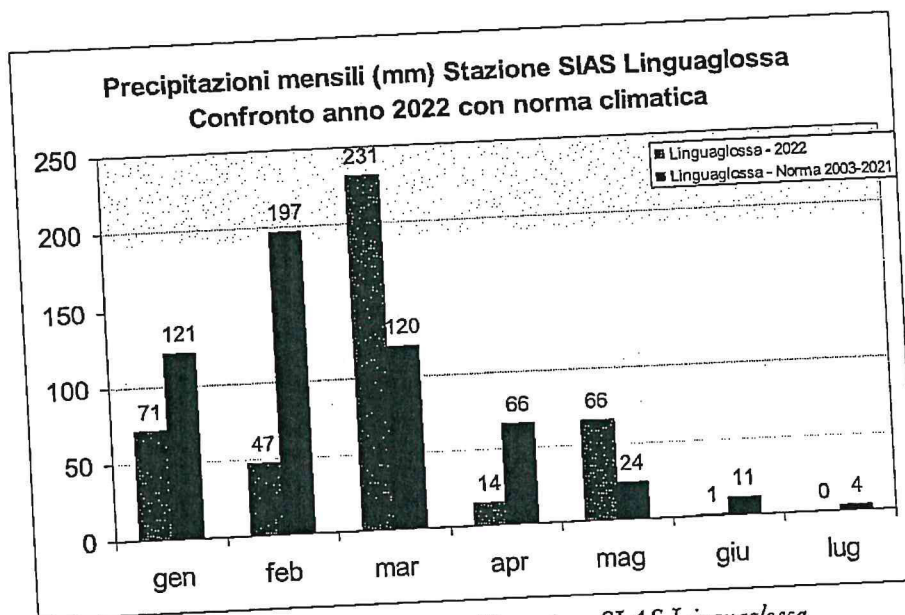
Grafico 4: Precipitazioni mensili stazione SIAS Linguaglossa
