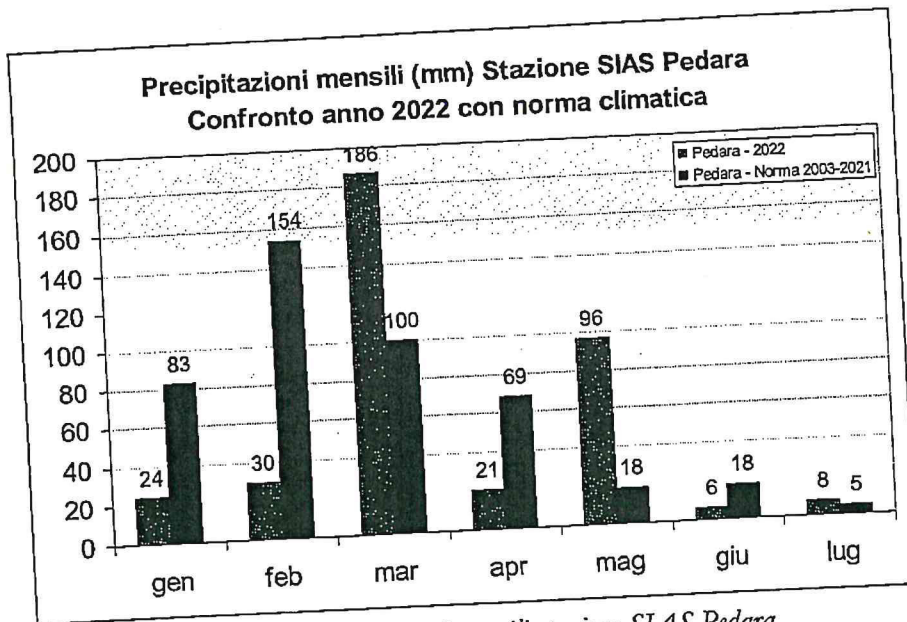
Grafico 9: Precipitazioni mensili stazione SIAS Pedara
