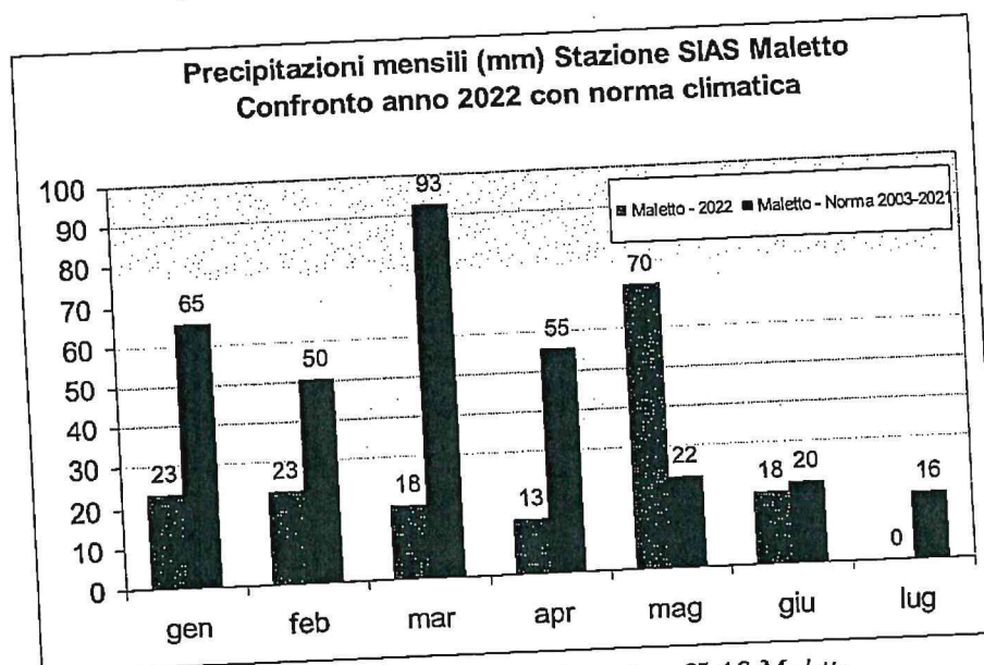
Grafico 5: Precipitazioni mensili stazione SIAS Maletto
