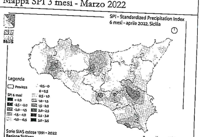
Mappa SPI 6 mesi - Aprile 2022
