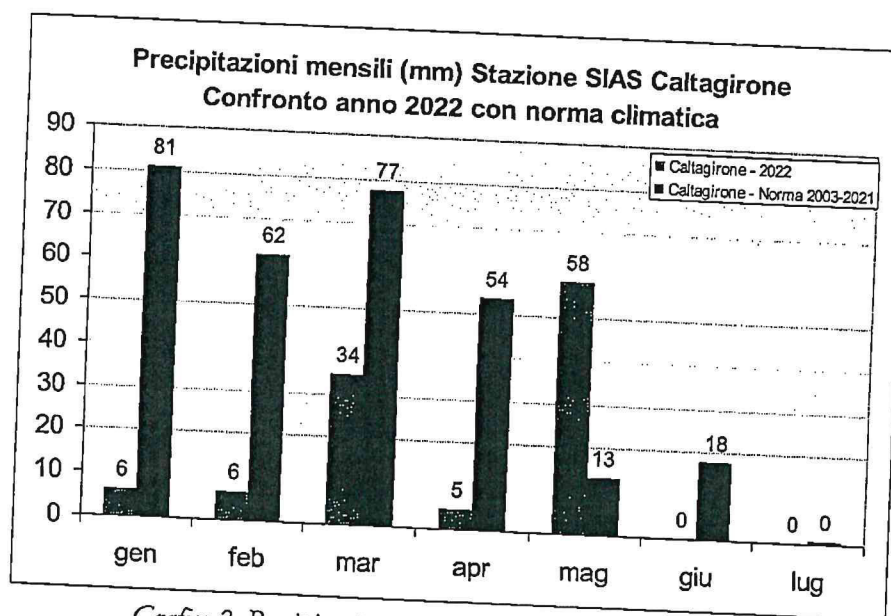
Grafico 2: Precipitazioni mensili stazione SIAS Caltagirone
