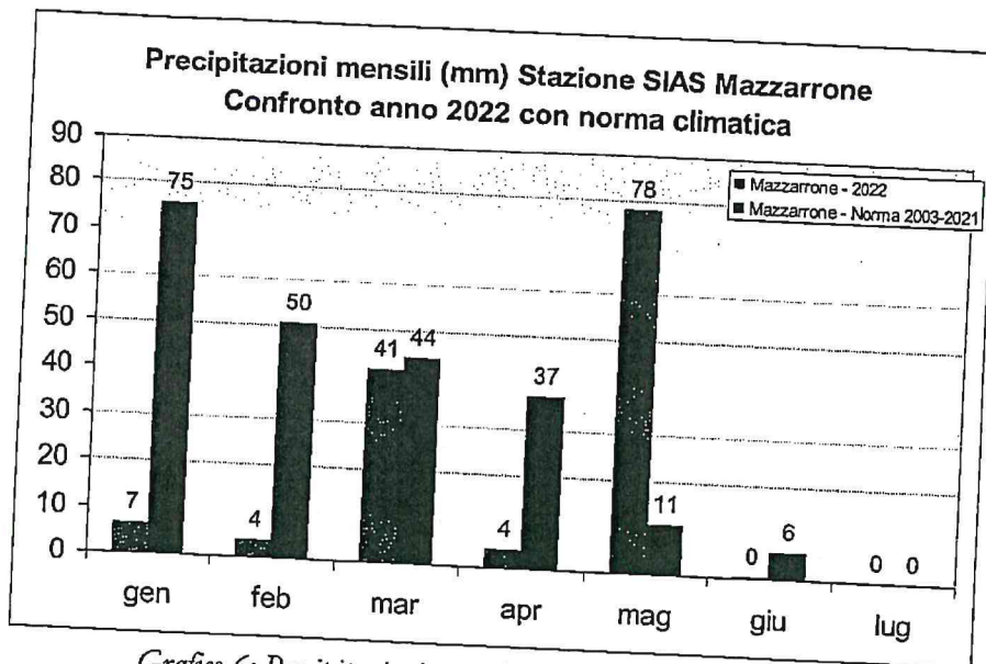
Grafico 6: Precipitazioni mensili stazione SIAS Mazzarrone
