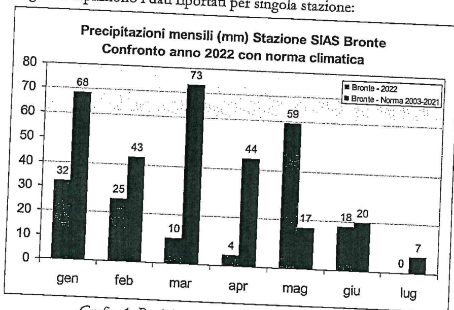
Grafico 1: Precipitazioni mensili stazione SIAS Bronte
