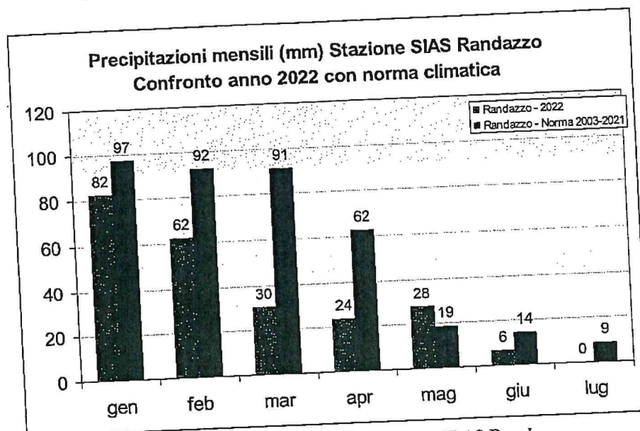
Grafico 11: Precipitazioni mensili stazione SIAS Randazzo
