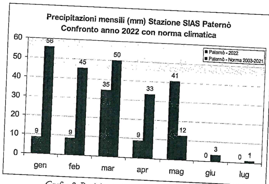
Grafico 8: Precipitazioni mensili stazione SIAS Paternò
