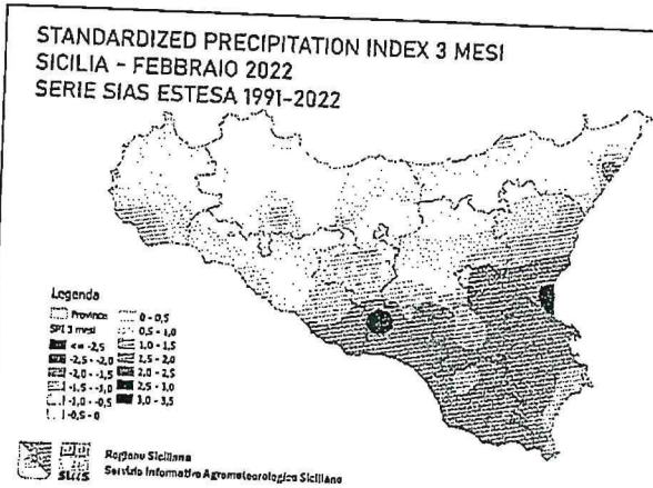
Mappa SPI 3 mesi - Febbraio 2022
