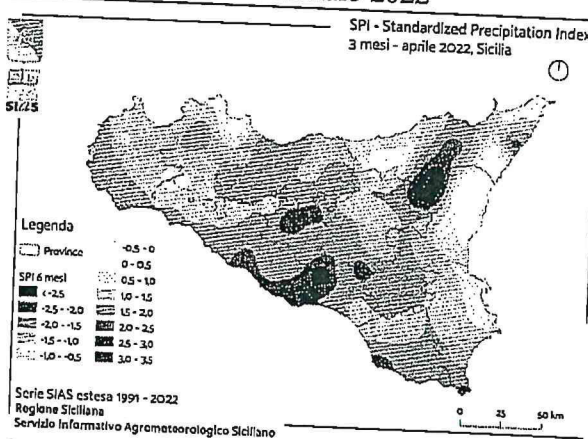
Mappa SPI 3 mesi - Aprile 2022
