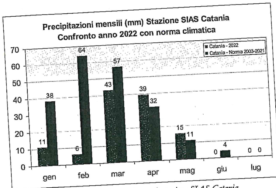
Grafico 3: Precipitazioni mensili stazione SIAS Catania
