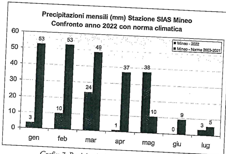
Grafico 7: Precipitazioni mensili stazione SIAS Mineo
