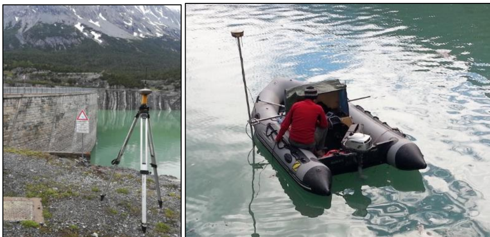
Figura 14-1: ricevitori GPS “base” posizionato a terra (a sinistra) e “rover” montato sul natante utilizzati per i rilievi morfobatimetrici (a destra)
