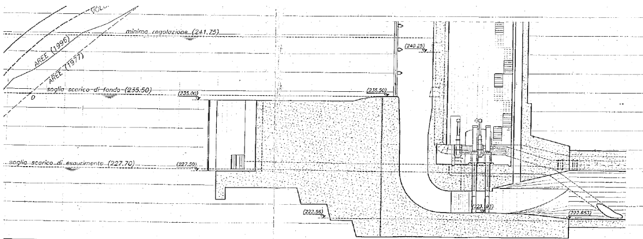
Figura 5-6: scarico di fondo e scarico di esaurimento della diga di Sciaguana
