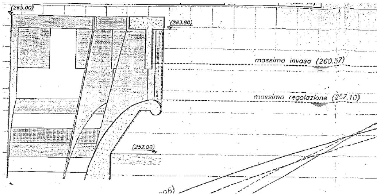
Figura 5-5: scarico di superficie della diga di Sciaguana
