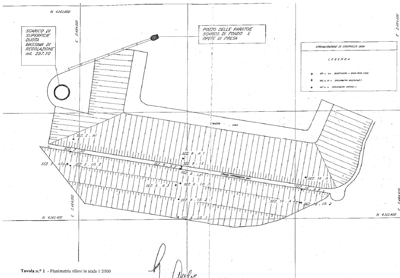
Figura 5-4: planimetria dello sbarramento di Sciacguana
