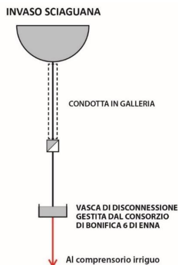
INVASO SCIAGUANA - SCHEMA IDRAULICO E UTILIZZO RISORSE
