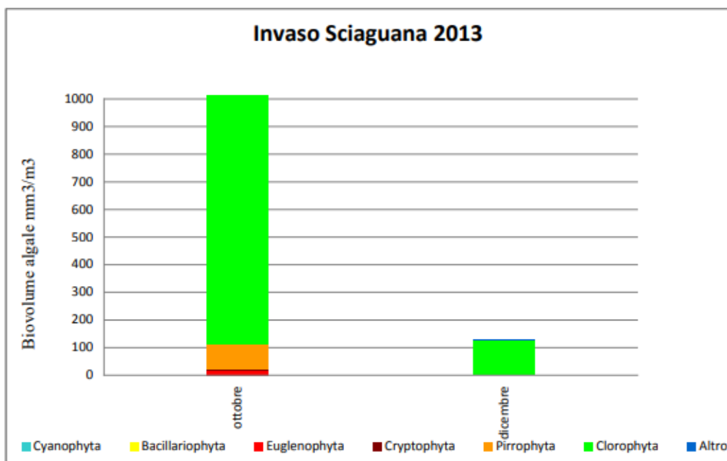
Figura 6-5: andamento abbondanza comunità fitoplanctonica (ARPA, 2013)
