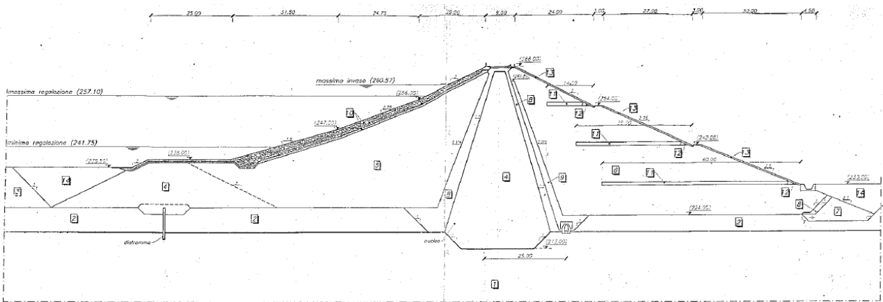
Figura 5-3: sezione trasversale della diga di Sciaguana
