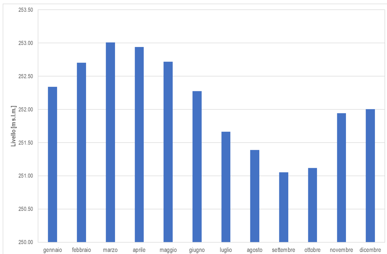
Figura 5-9: andamento dei livelli del bacino di Sciaguana
