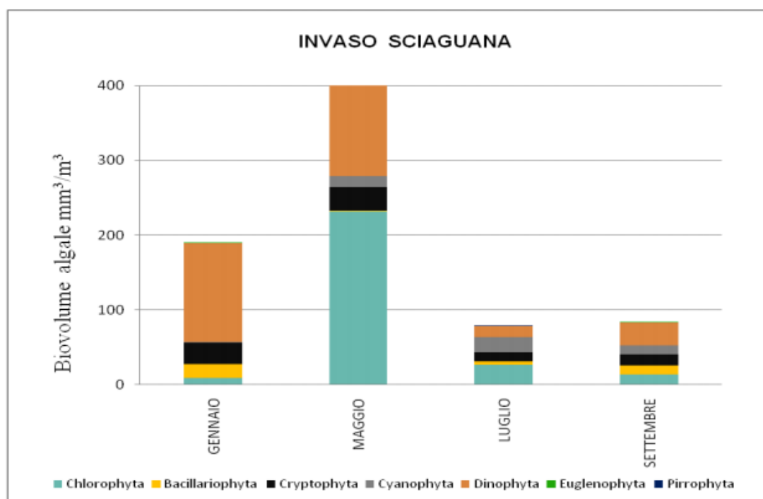
Figura 6-6: andamento abbondanza comunità fitoplanctonica (ARPA, 2014)
