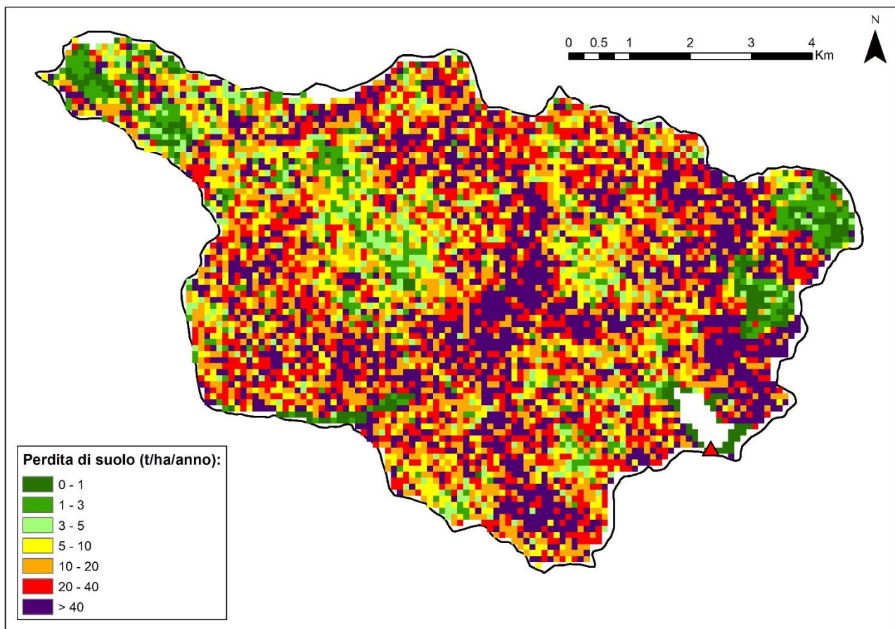
Figura 5-10: elaborazione RUSLE del bacino imbrifero diretto sotteso dalla diga di Sciaguana (indicata dal triangolo rosso)
