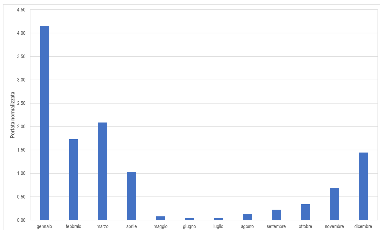
Figura 5-8: portate normalizzate del F. Simeto a Biscari (fonte: PTA Sicilia)
