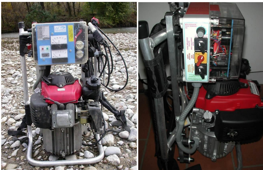
Figura 14-11: elettroscandaglio spallabile da 1300 W
