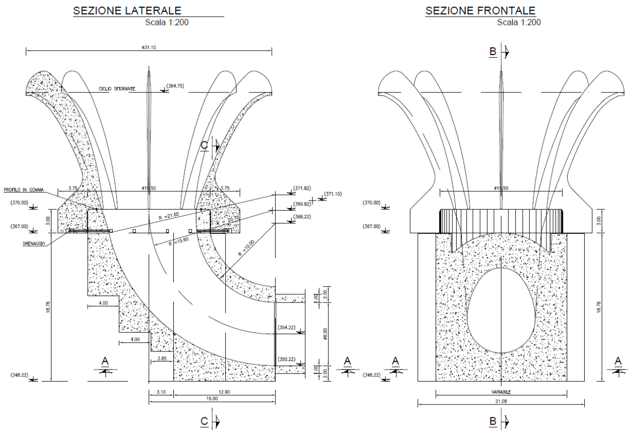
Figura 5-5: scarico di superficie della diga di Nicoletti
