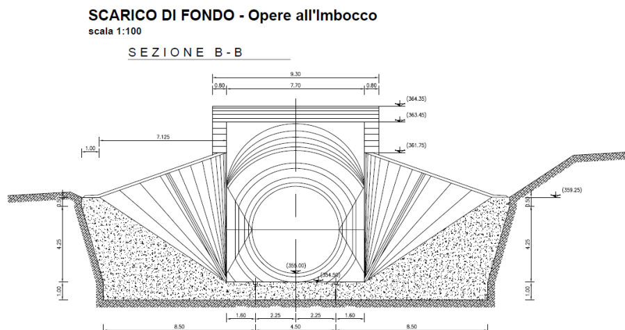
Figura 5-7: scarico di fondo della diga di Nicoletti
