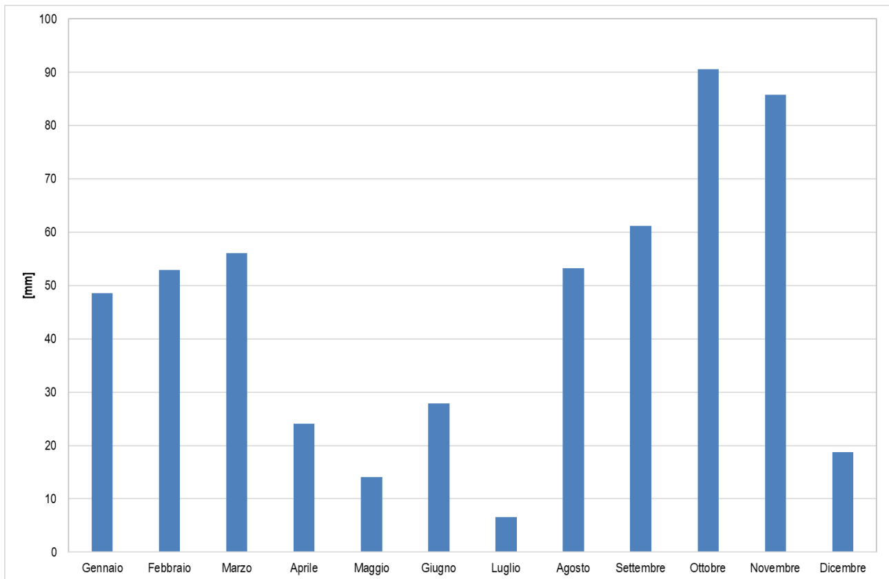
Figura 3-6: pioggia cumulata media mensile (periodo 2015-2020)
