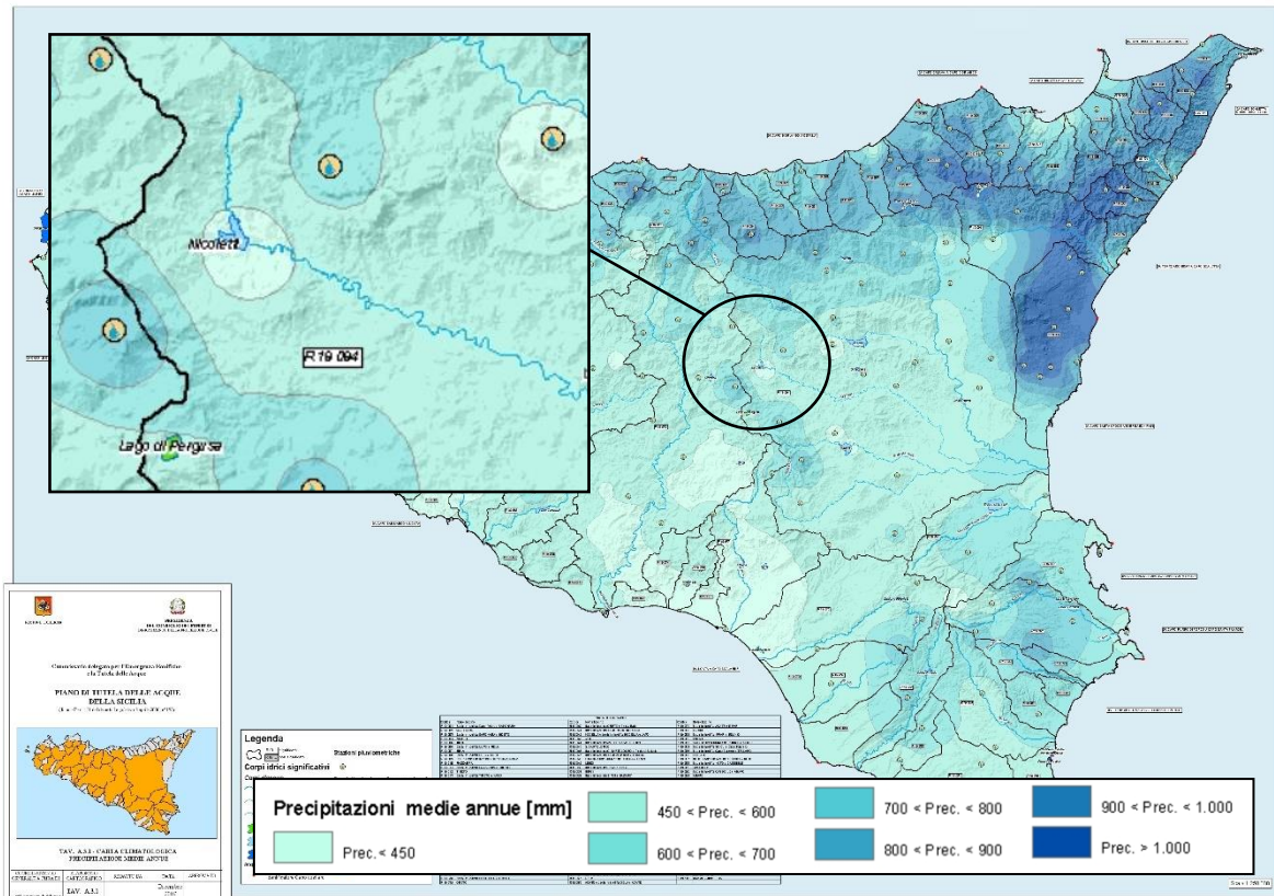
Figura 3-7: estratto della tavola A.3.1 “Carta climatologica – Precipitazioni medie annue” del PTA
