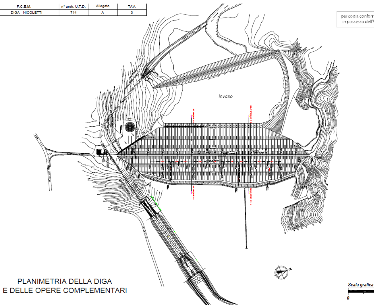
Figura 5-4: planimetria dello sbarramento di Nicoletti
