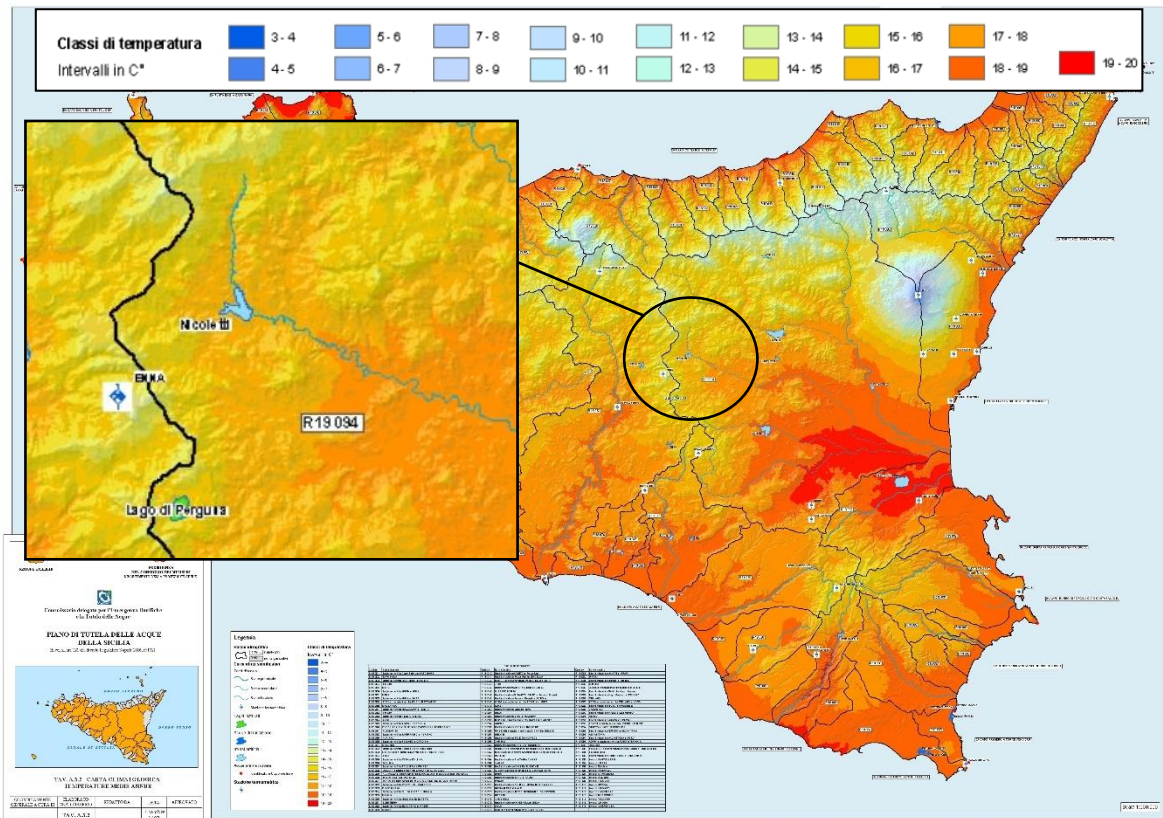
Figura 3-8: estratto della tavola A.3.2 “Carta climatologica – Temperature medie annue” del PTA
