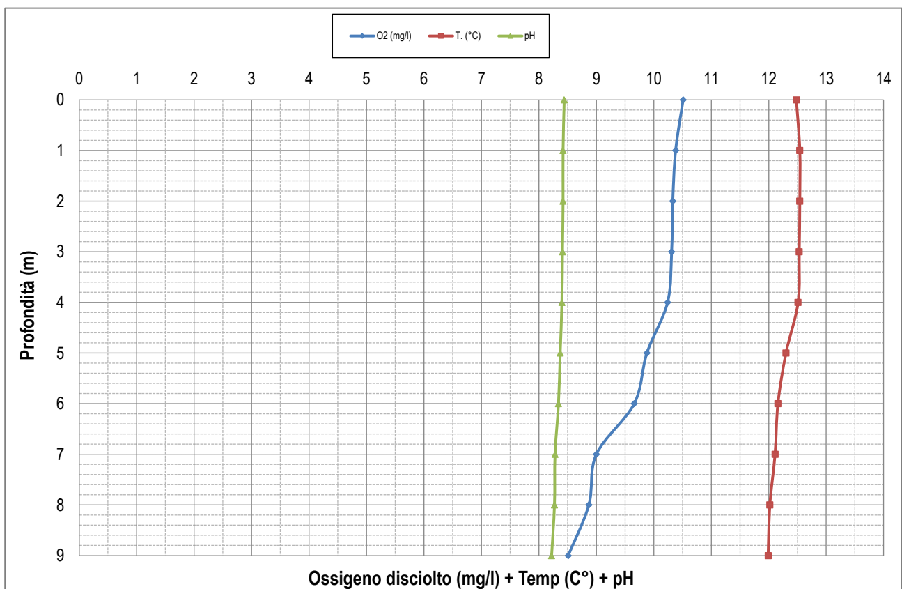
Figura 6-4: confronto degli andamenti di ossigeno disciolto, temperatura e pH sulla colonna d'acqua
