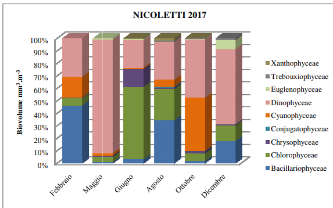
Figura 6-5: andamento abbondanza comunità fitoplanctonica (ARPA, 2017)
