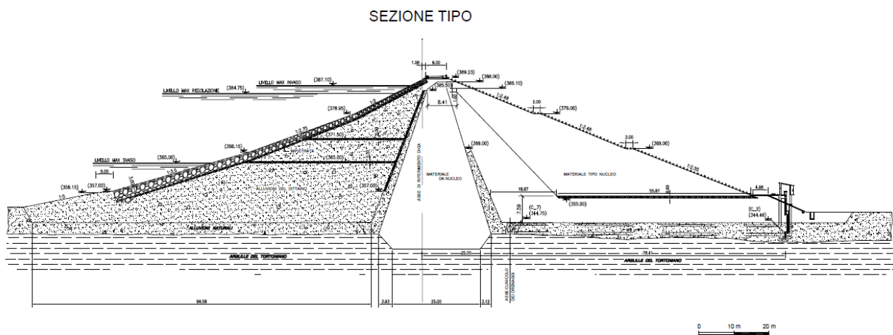
Figura 5-3: sezione tipo della diga di Nicoletti
