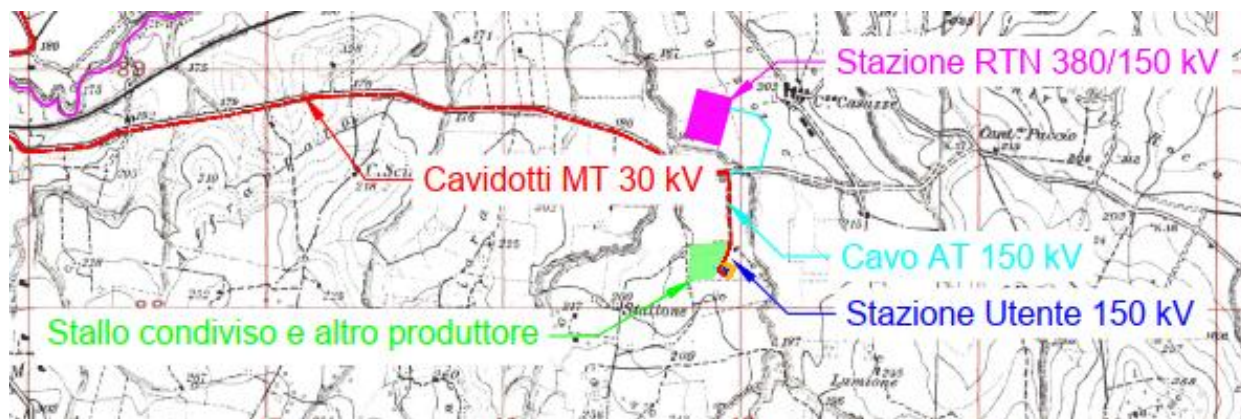
Figura 2 – Opere di connessione e di rete - Estratto di inquadramento generale da IGM
