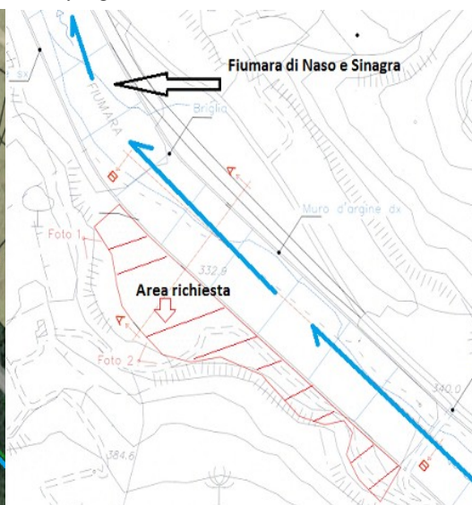
Stralcio Aerofotogrammetria
