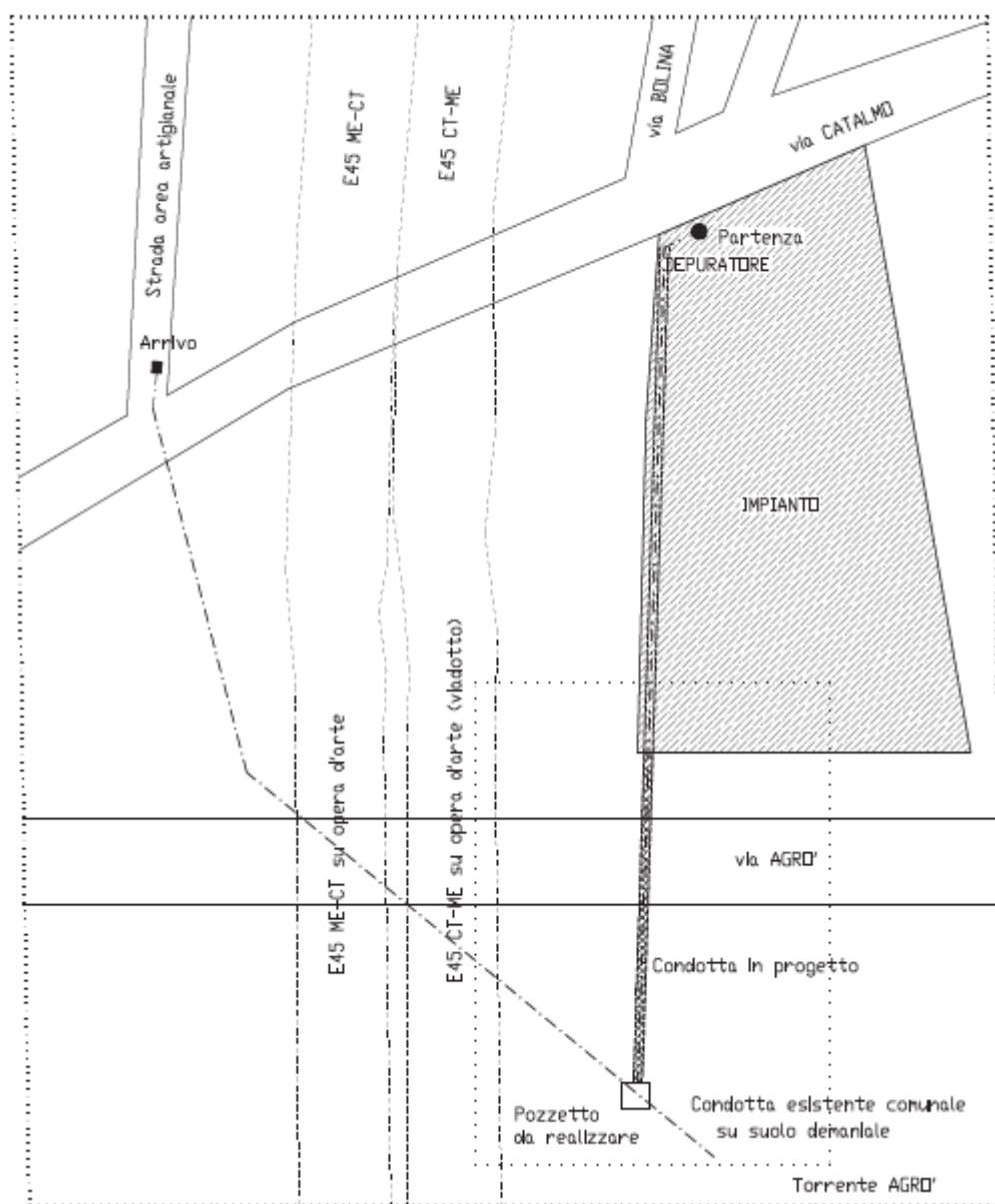
Planimetria Generale 1500
