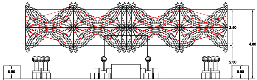
A-A posizionamento luminarie h 2.3
