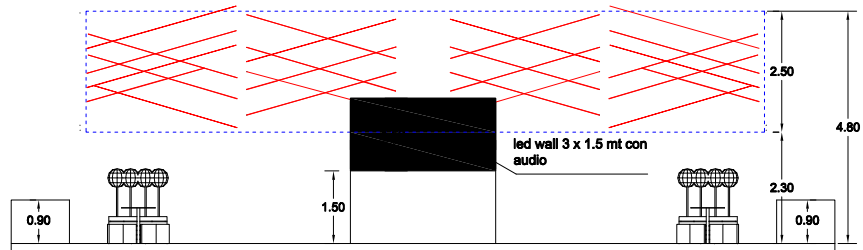
B-B posizionamento vele tra h 2.3 e h 4.8
