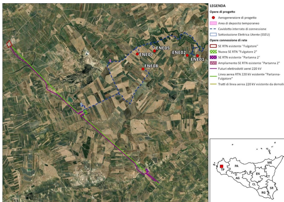
Figura 1.2: Inquadramento dell'impianto in variante comprensivo delle opere connesse
