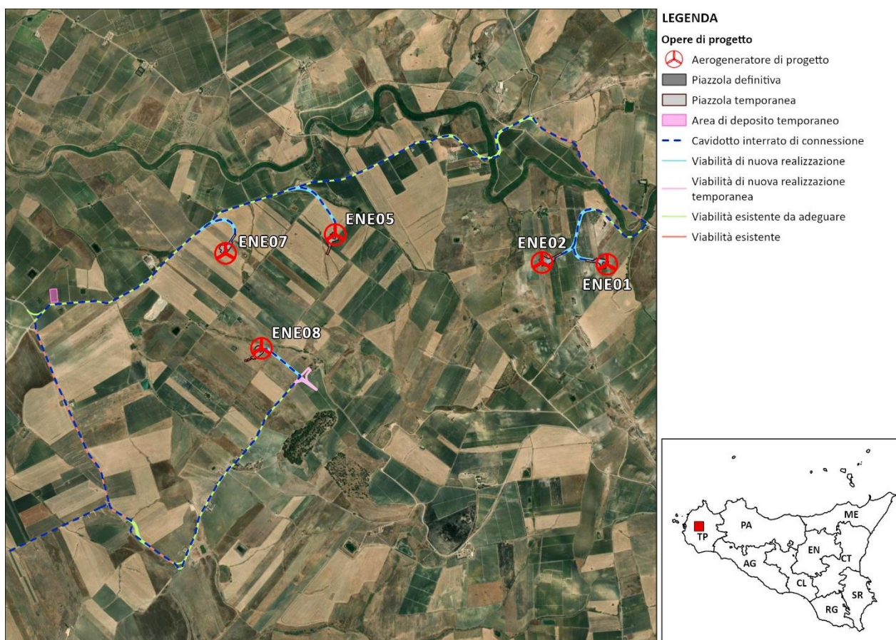
Figura 1.3: Inquadramento della viabilità di progetto
