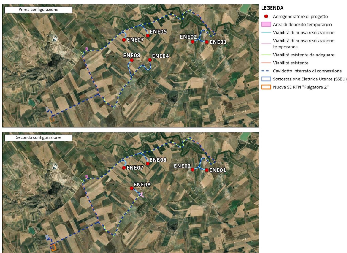
Figura 1.1: Confronto fra la prima e la seconda configurazione
