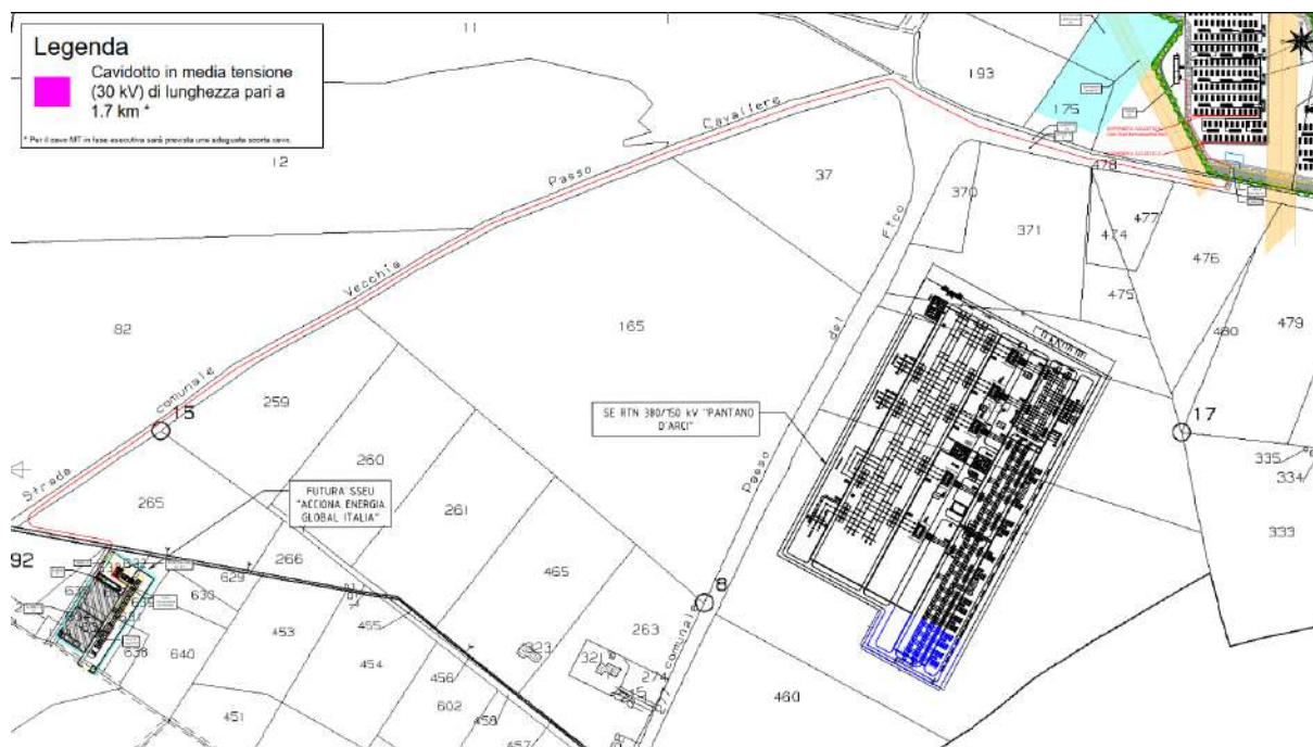
Figura 1: Inquadramento catastale elettrodotto
