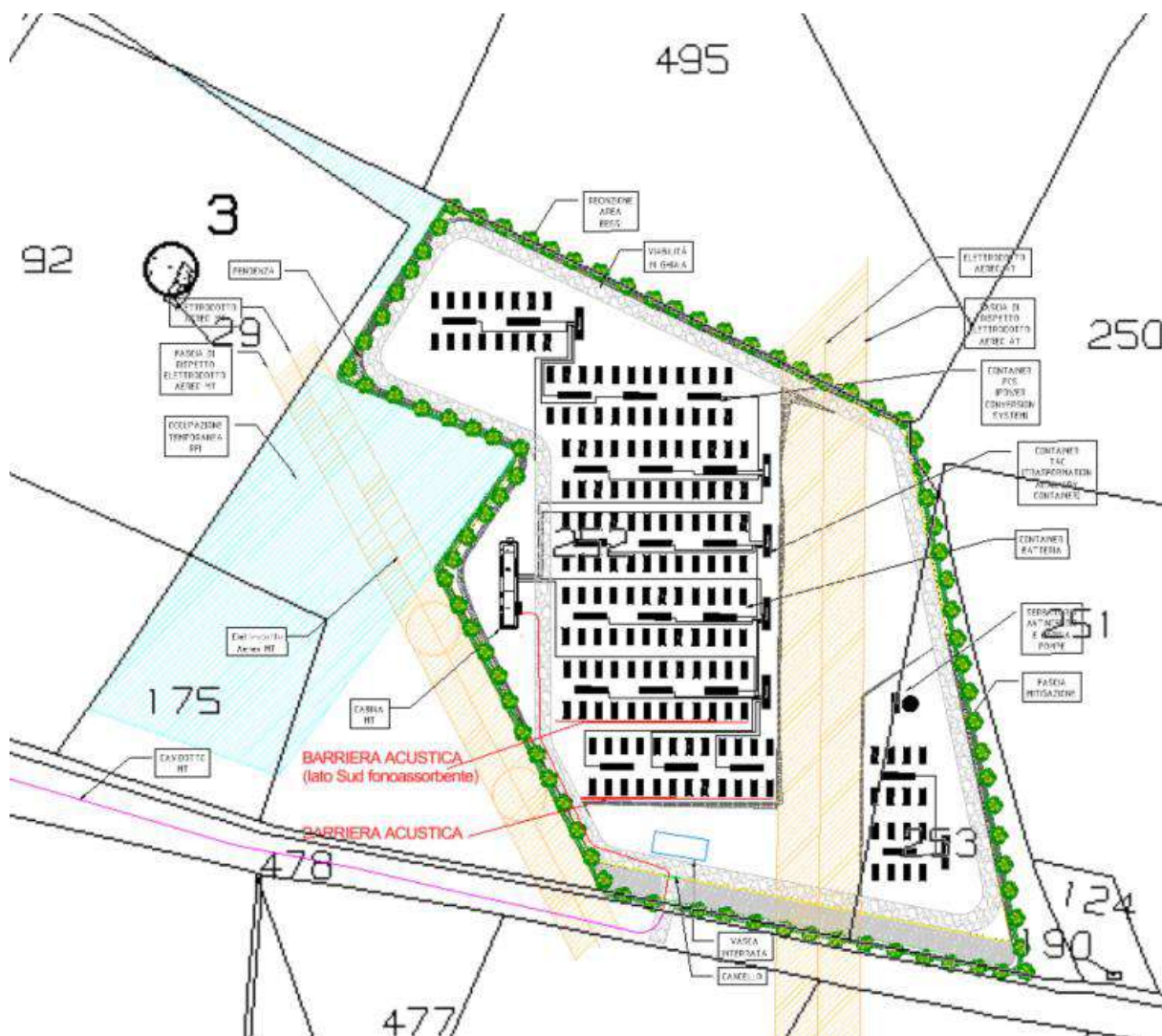
Figura 2: Inquadramento catastale impianto BESS
