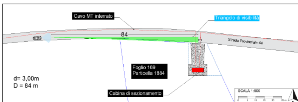
Figura 8 – Costruzione triangolo visibilità
