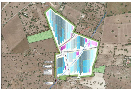
Figura 1 – Layout di Impianto AGV Crucetta
