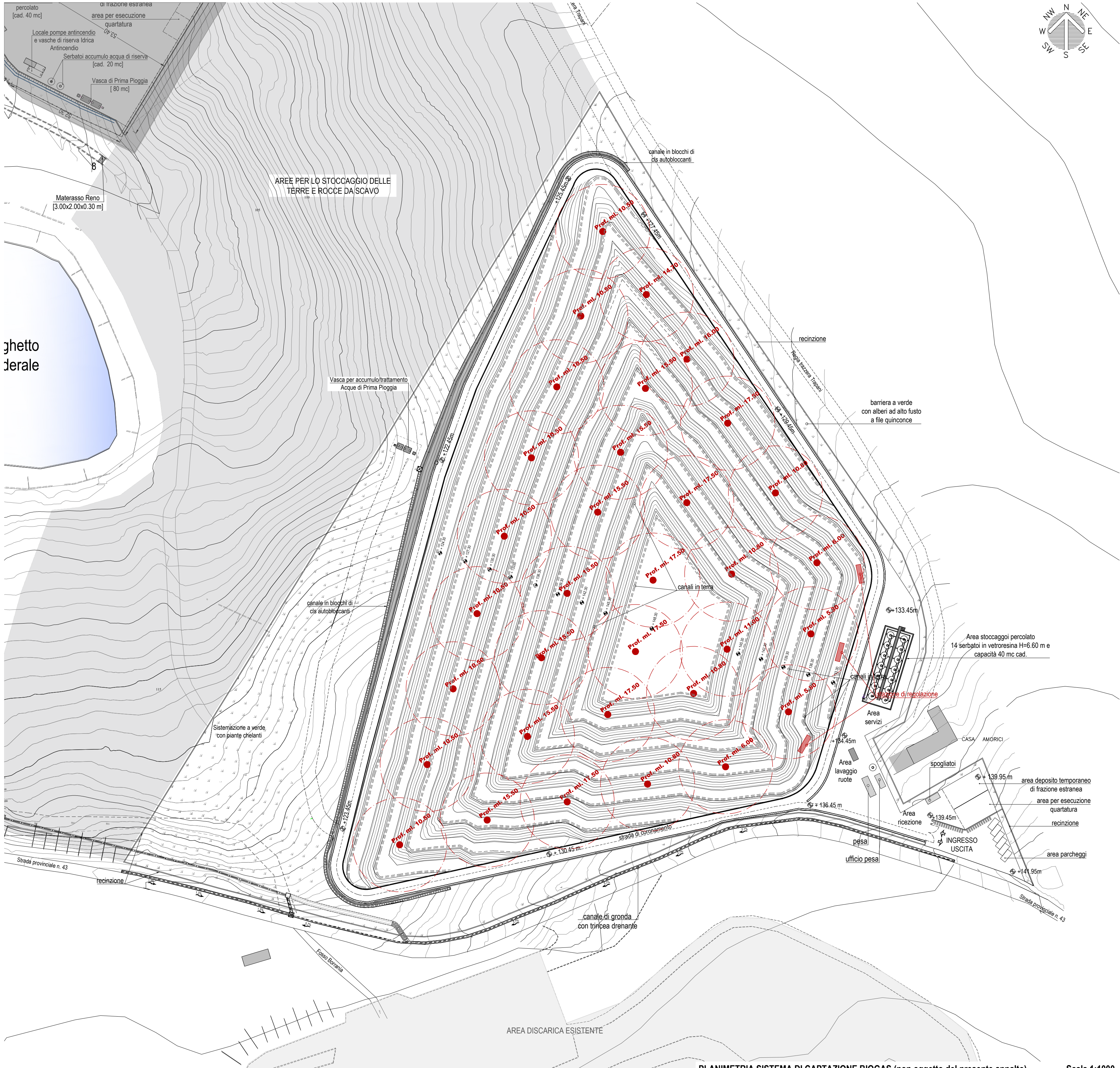
PLANIMETRIA SISTEMA DI CAPTAZIONE BIOGAS (non oggetto del presente appalto) Scala 1:1000 (quote espresse in metri)
