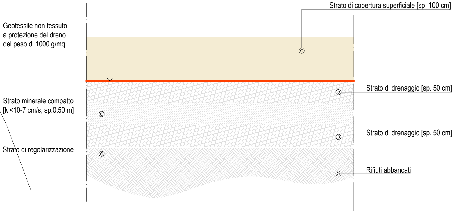
PACCHETTO CAPPING Scala 1:50
