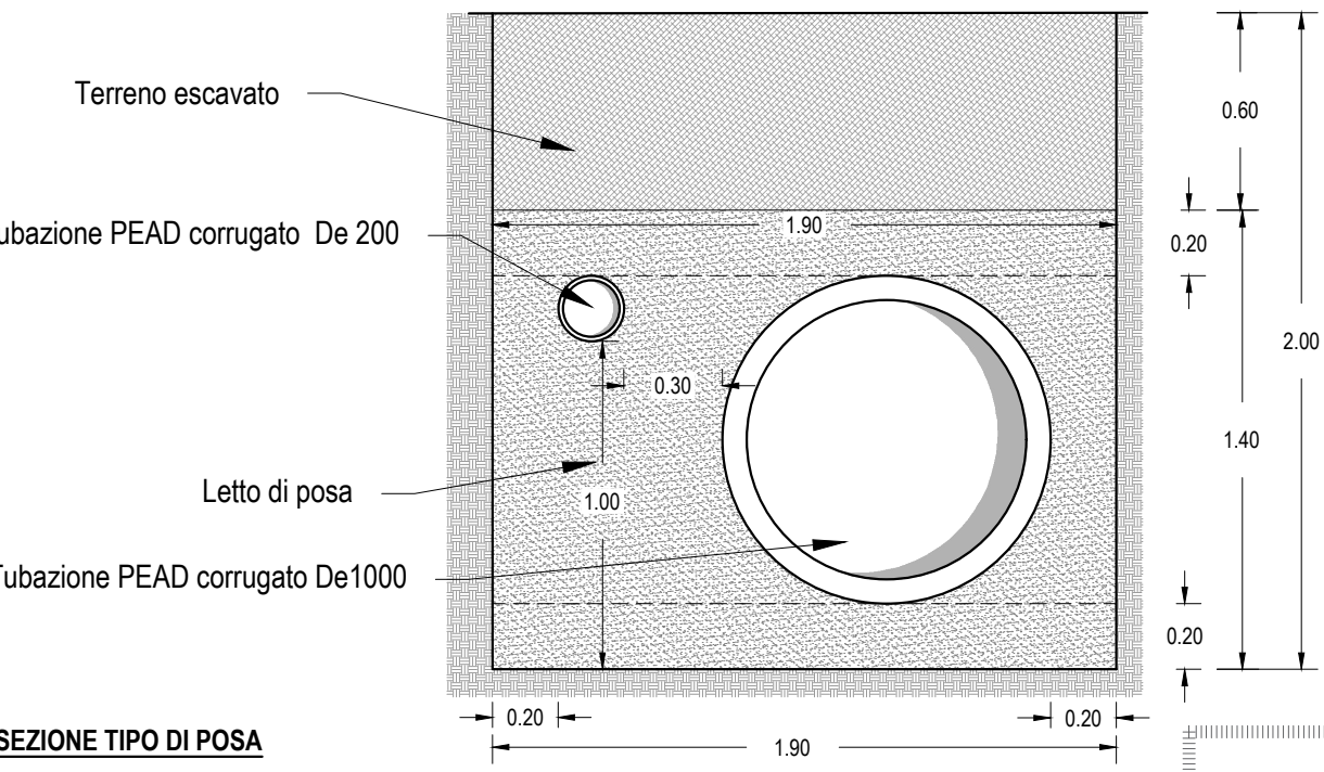
SEZIONE TIPO E PARTICOLARE AREA DI RECAPITO LINEA DI TRASPORTO ACQUE BIANCHE scala 1:25
