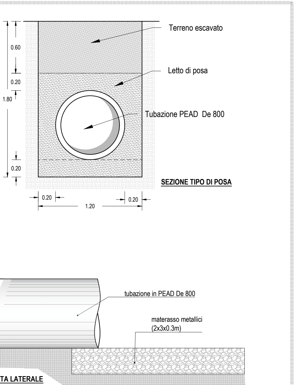
SEZIONE TIPO E PARTICOLARE AREA DI RECAPITO DELLA CONDOTTA DI ALLONTANAMENTO PEAD De 800 scala 1:25
