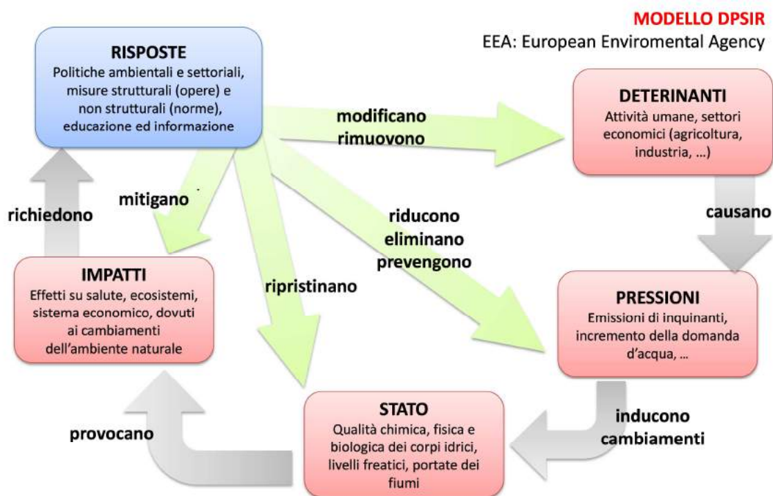
Figura 6.2: Modello DPSIR
