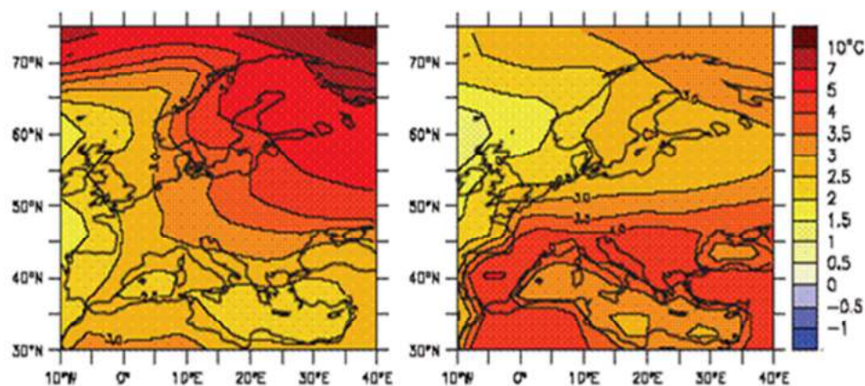
Figura 3.3: Variazione della temperatura media in Europa dal 1980-1999 e dal 2009-2099, stimata sulla base dello scenario di emissione A1B
