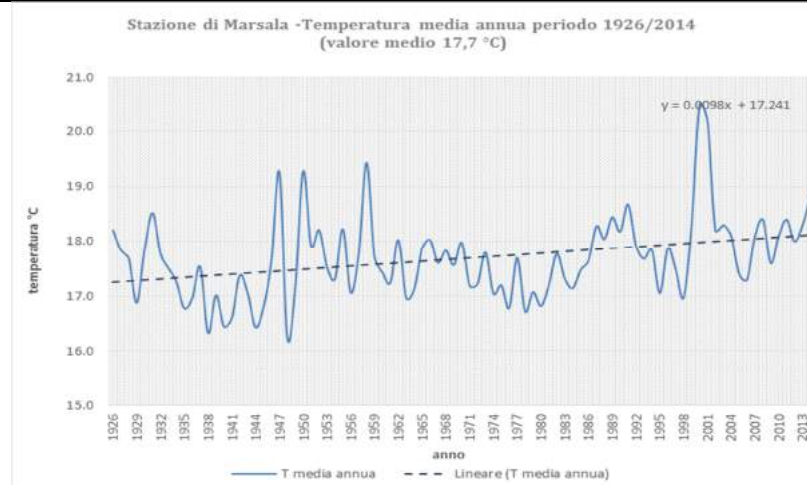
Figura 3.13: Stazione di Marsala – Temperatura media annua periodo 1926-2014
