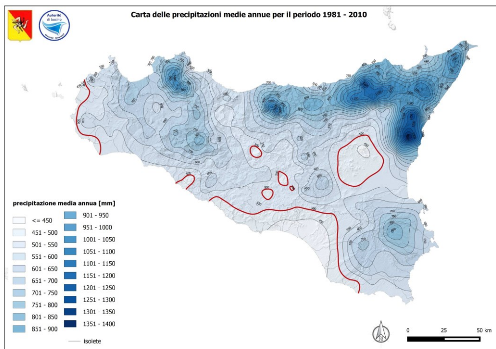
Figura 3e – carta delle isoiete per il trentennio 1981-2010.
