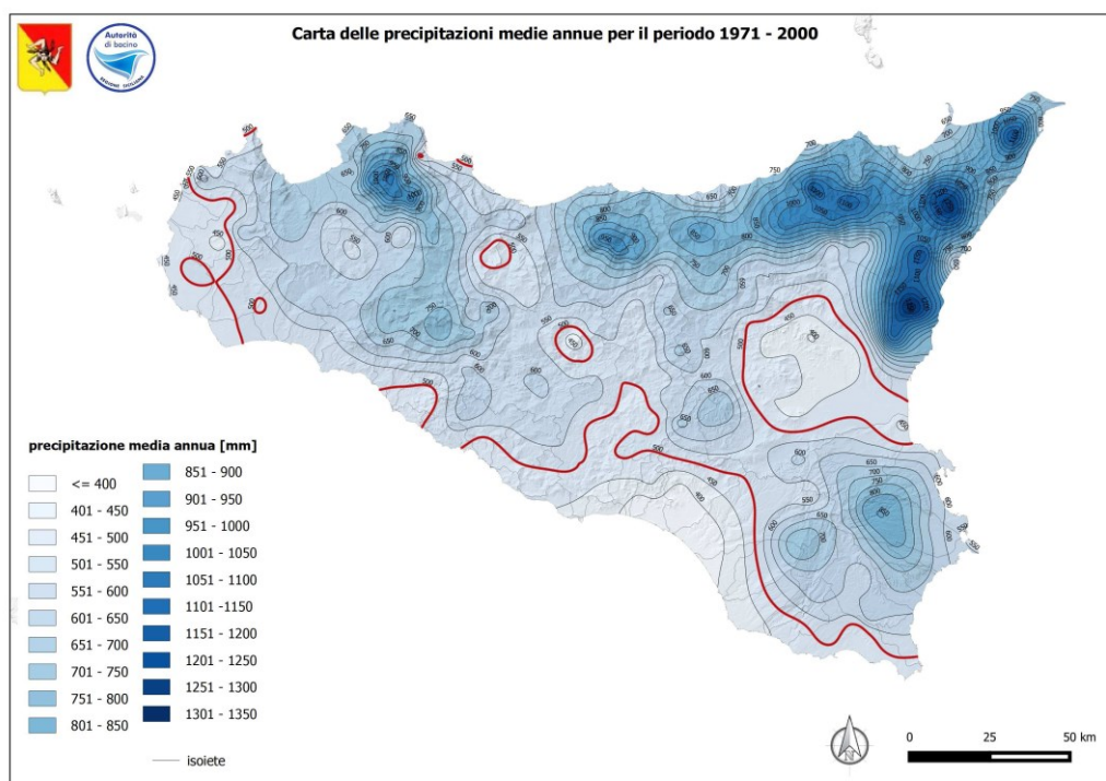
Figura 3d – carta delle isoiete per il trentennio 1971-2000.
