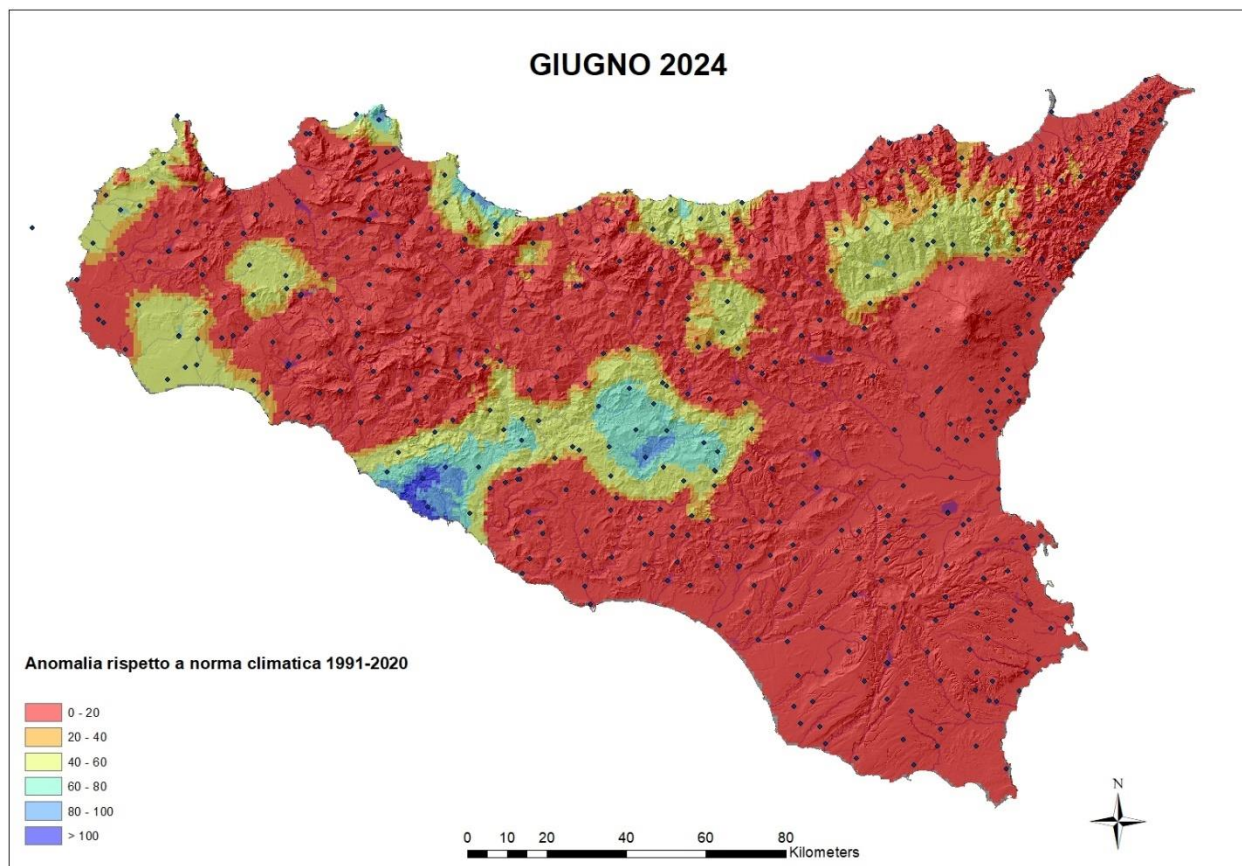
Fig. 2 – anomalia di precipitazione giugno 2024 / giugno 1991-2020
