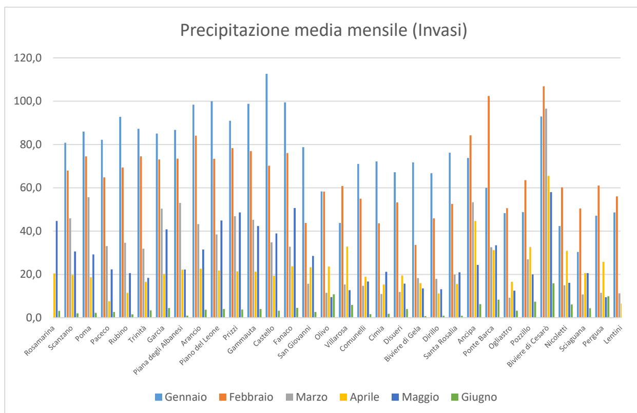
Fig. 5 – precipitazione mensile giugno 2024 ai bacini sottesi agli sbarramenti
