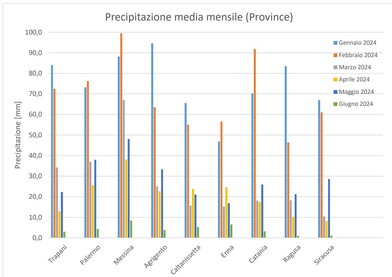
Fig. 4 – precipitazione mensile giugno 2024 a livello provinciale
