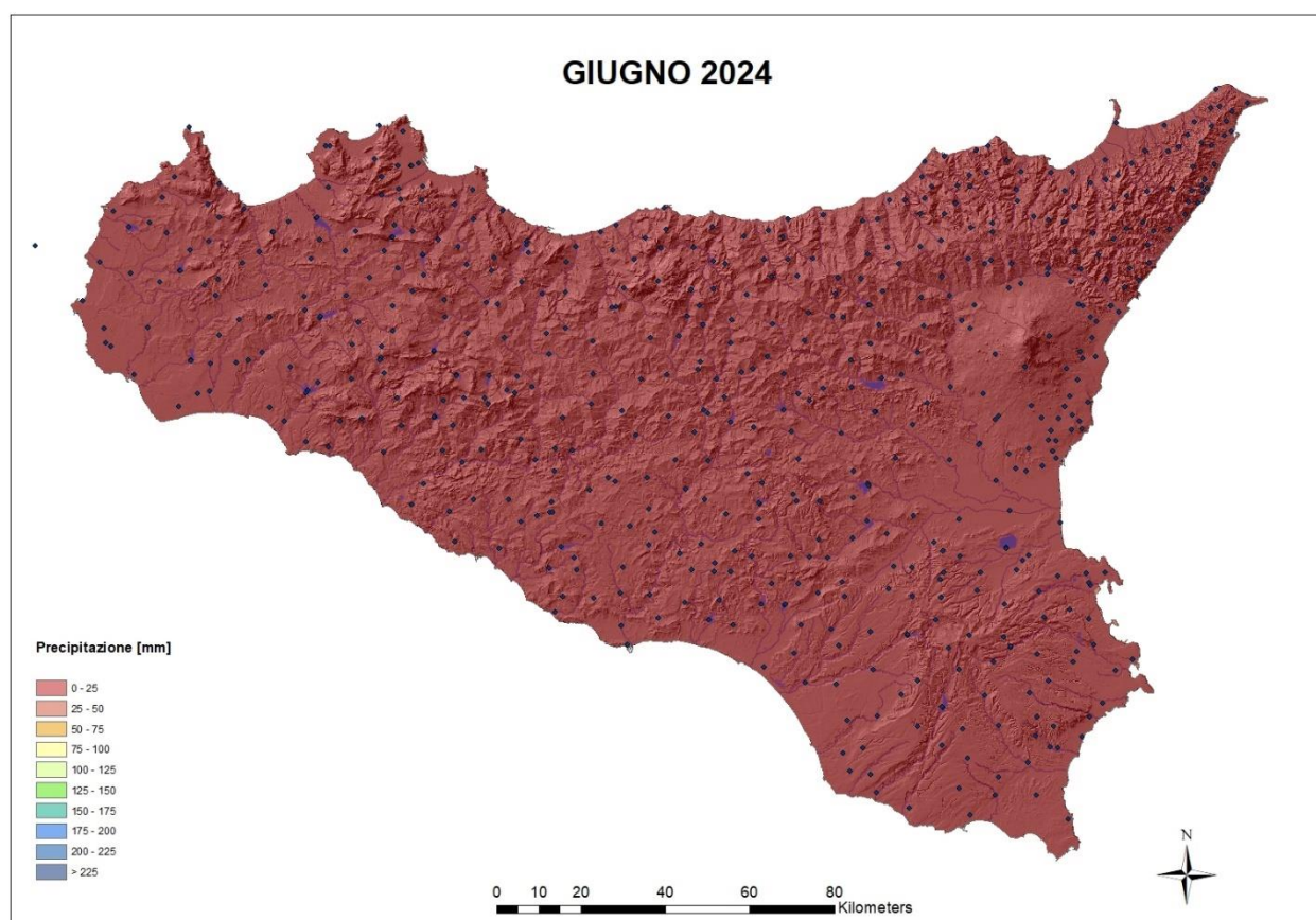
Fig. 1 – precipitazione media mensile di giugno 2024
