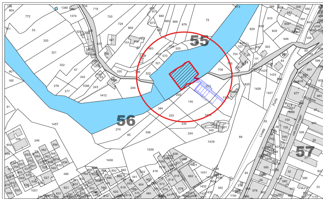
Figura 2: Stralcio mappa catastale porzioni del torrente comprese tra Foglio 55 particelle 320, 321, 570 e foglio 56 particelle 200 e 212 in Territorio del Comune di Scicli (RG)
